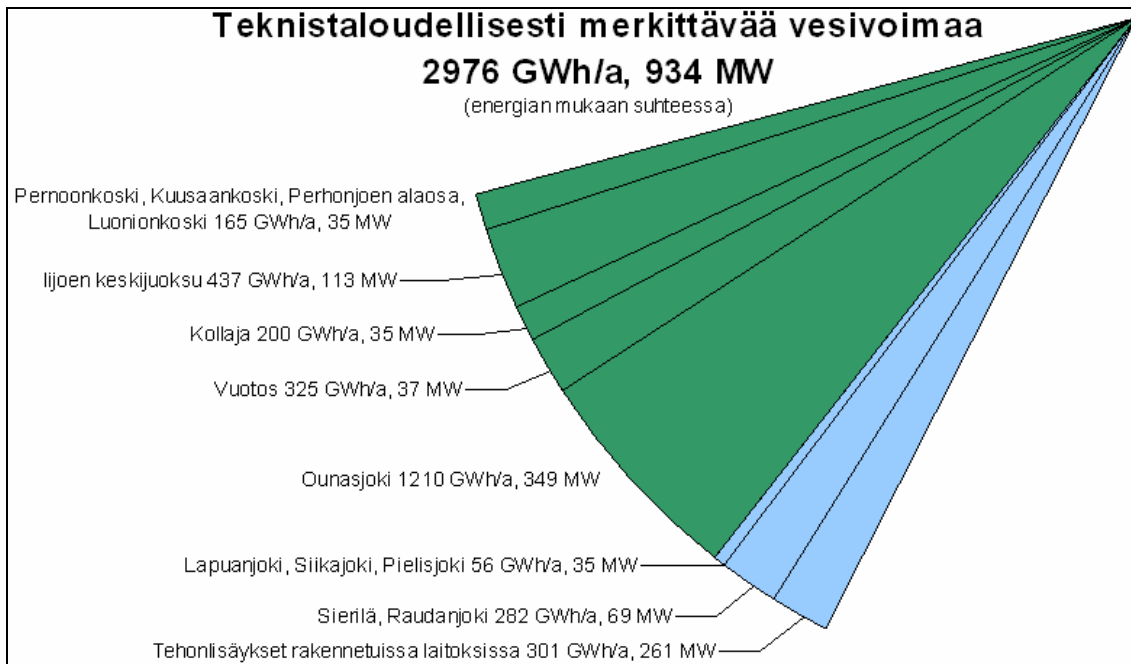
Teknistaloudellisesti merkittävä vesivoima energiamäärän mukaan, vihreällä suojelun alaiset kohdet (Oy Vesirakentaja 2008).
